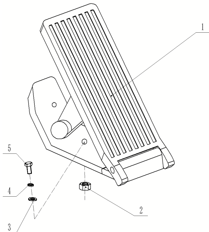
MTF25/30-45E, MTF25/30-60E
